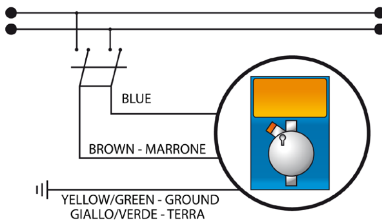
Fig.3 – Conexão elétrica
